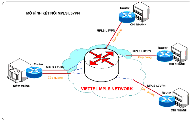
Hình 1: Mô hình kết nối giữa các điểm chi nhánh và điểm chính
